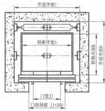
井道平面图 (砖混)
