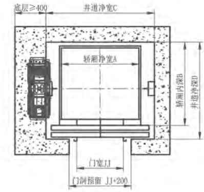
井道平面图 (砖混)
