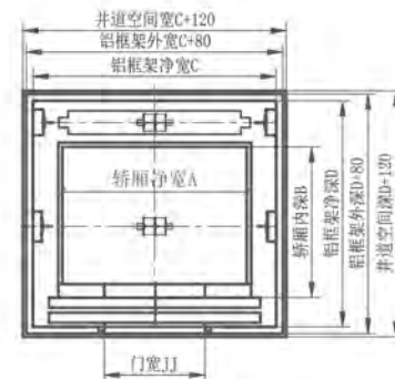
井道平面图 (铝型材)
