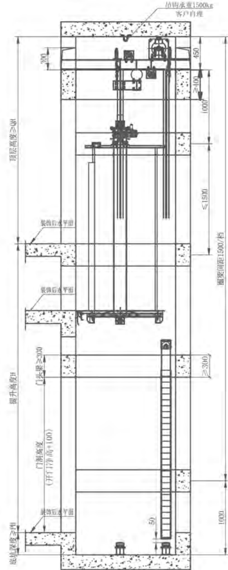
井道立面图
