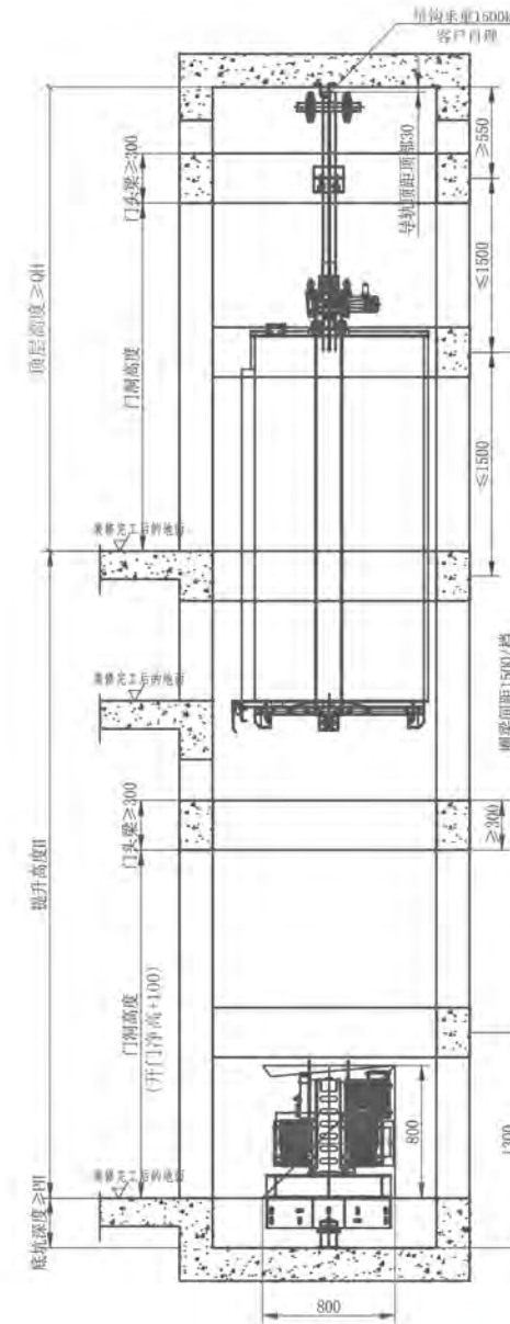
井道立面图
